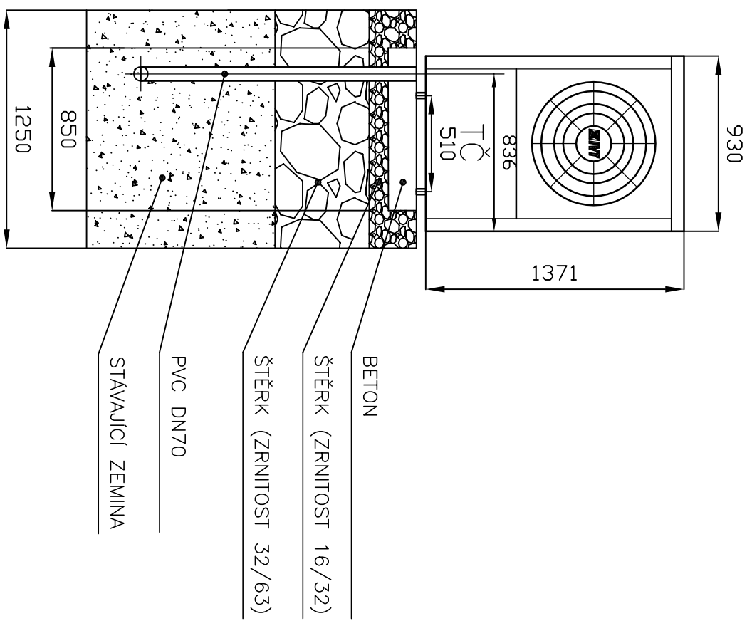
ČELNÍ POHLED
