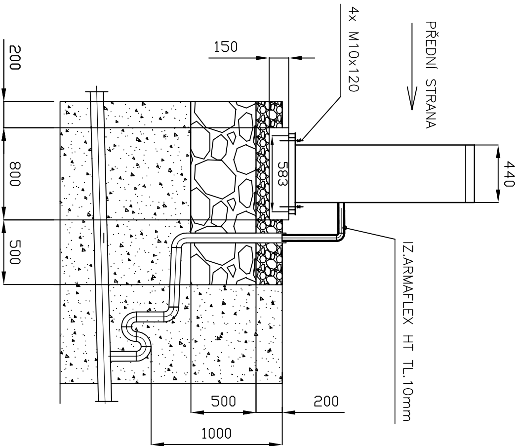
BOČNÍ POHLED
